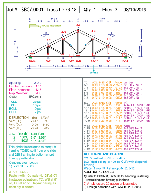
EXAMPLE OF A TRUSS DESIGN DRAWING EJEMPLO DE UN DIBUJO DEL DISEÑO DE TRUSSES
